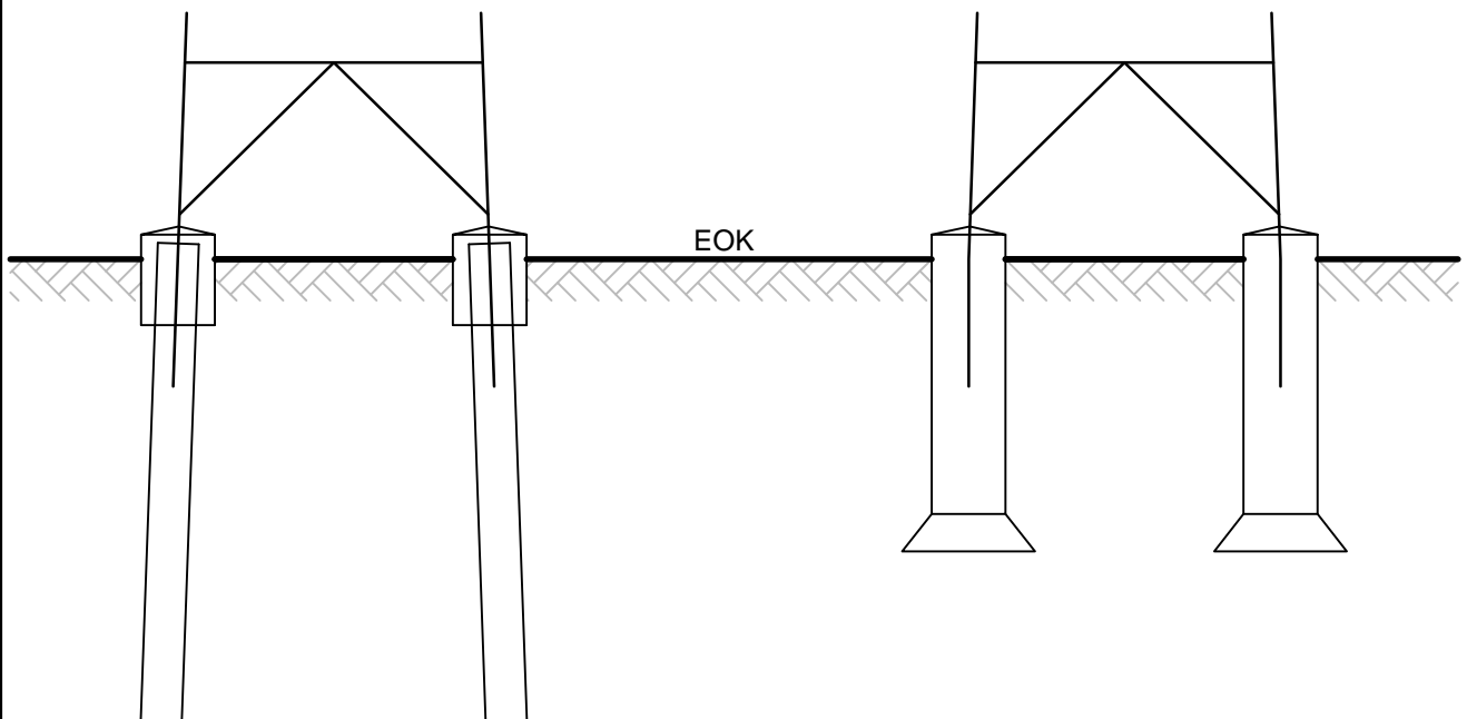
Rammpfahlfundament
