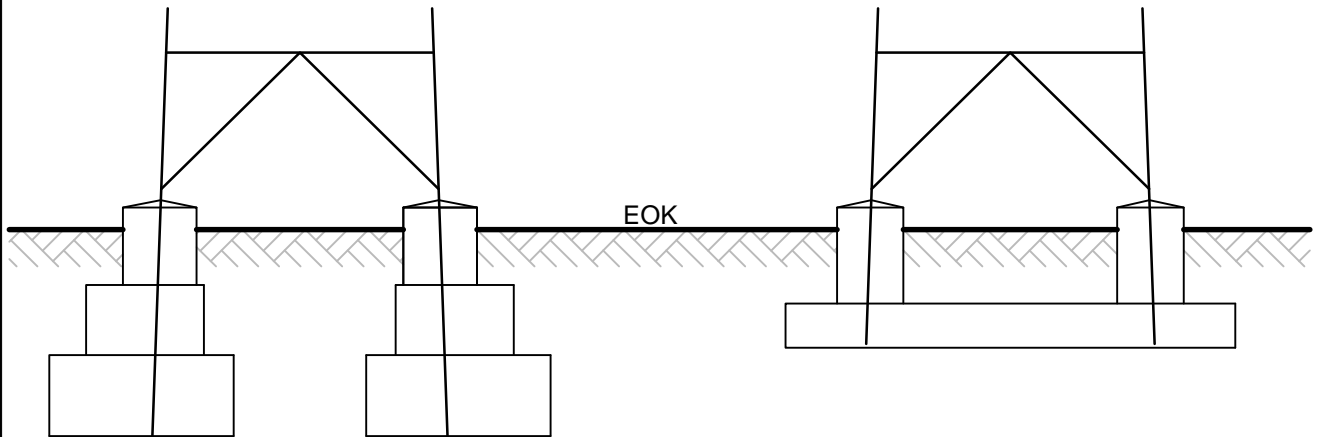
Stufenfundament
