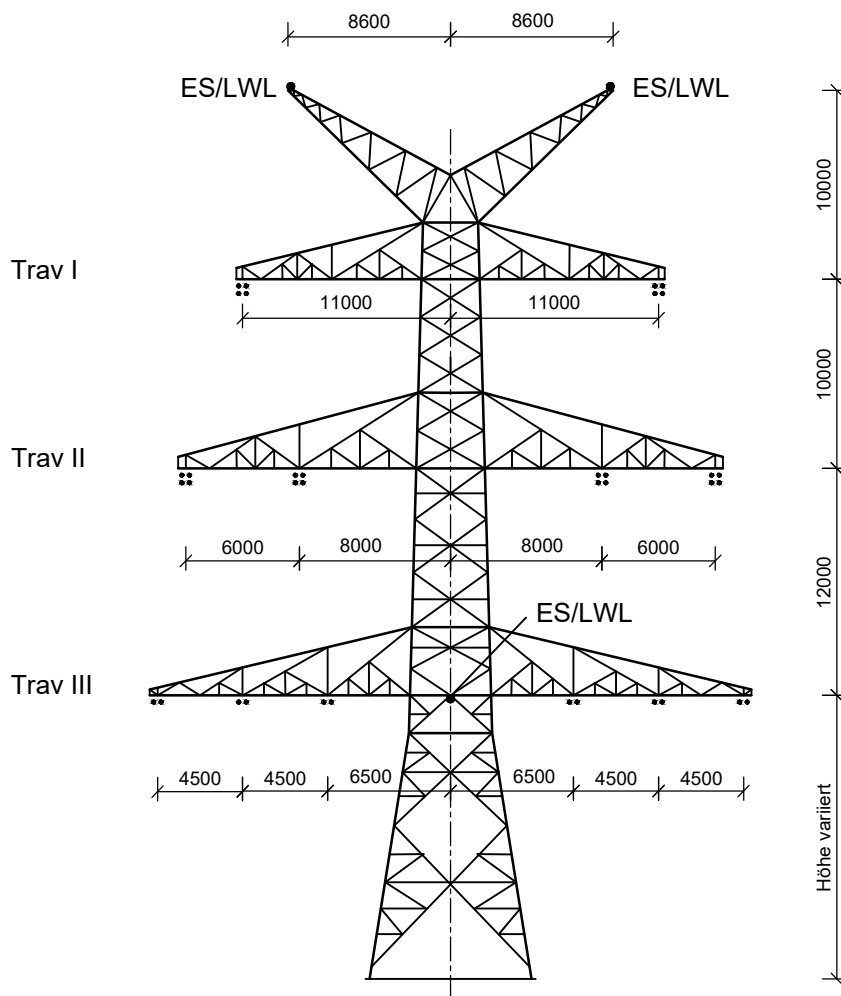
Winkelabspannmast WA160 ; DA-4-DE Ltg. Nr. B159: Mast-Nr. 117, 118, 122, 123
