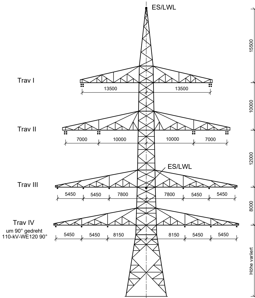
Winkelabspannmast WA120WAZ ; DA-4-DE Ltg. Nr. B159: Mast-Nr. 79
