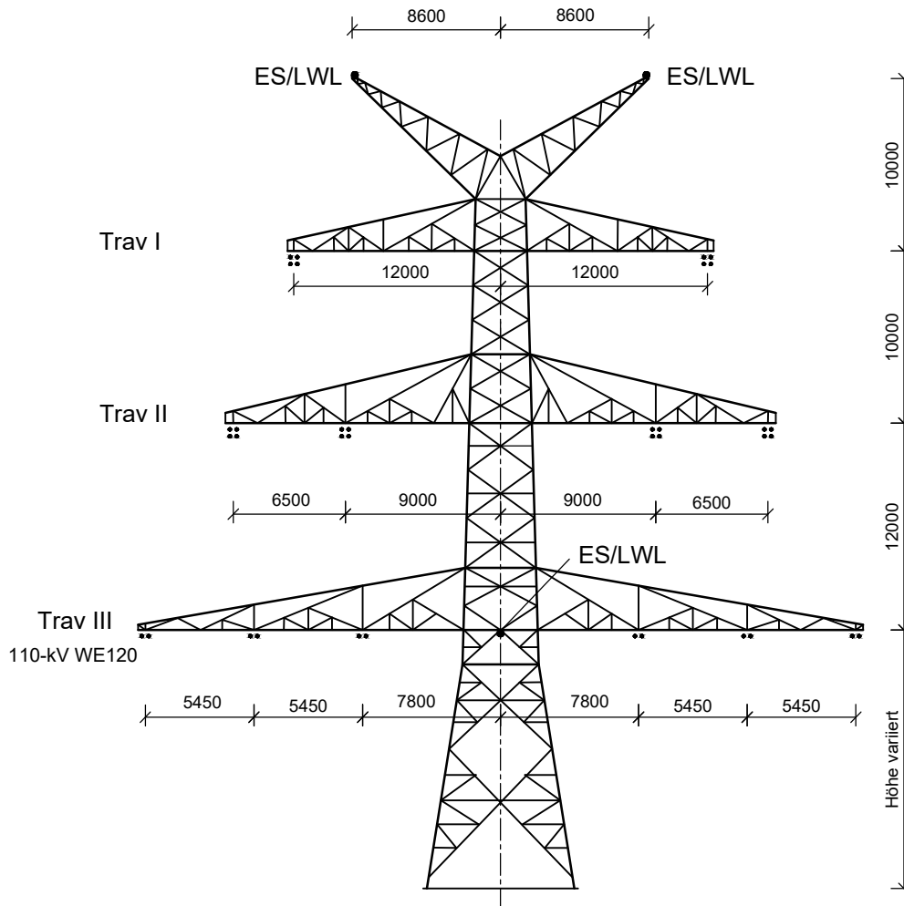
Winkelabspannmast WA140WAZ ; DA-4-DE Ltg. Nr. B159: Mast-Nr. 111,108
