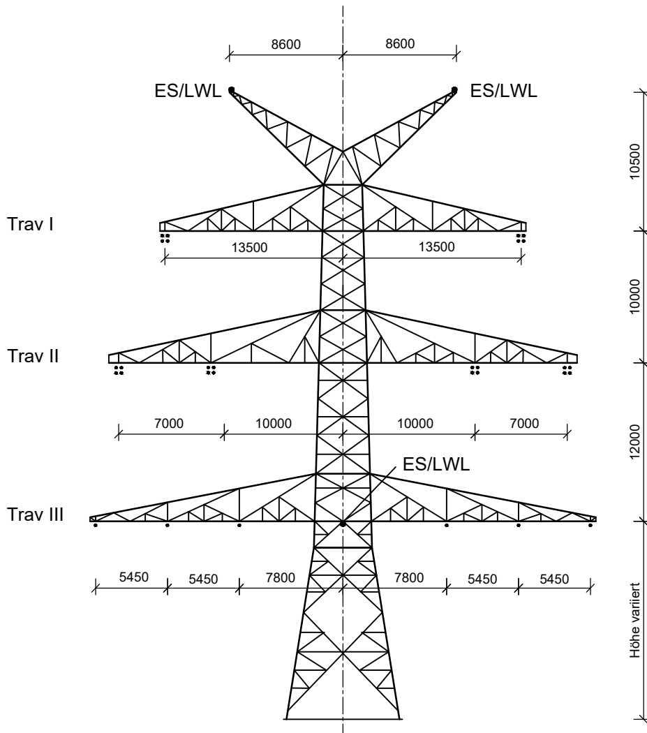
Winkelabspannmast WA120 ; DA-4-DE Ltg. Nr. B159: Mast-Nr. 115
