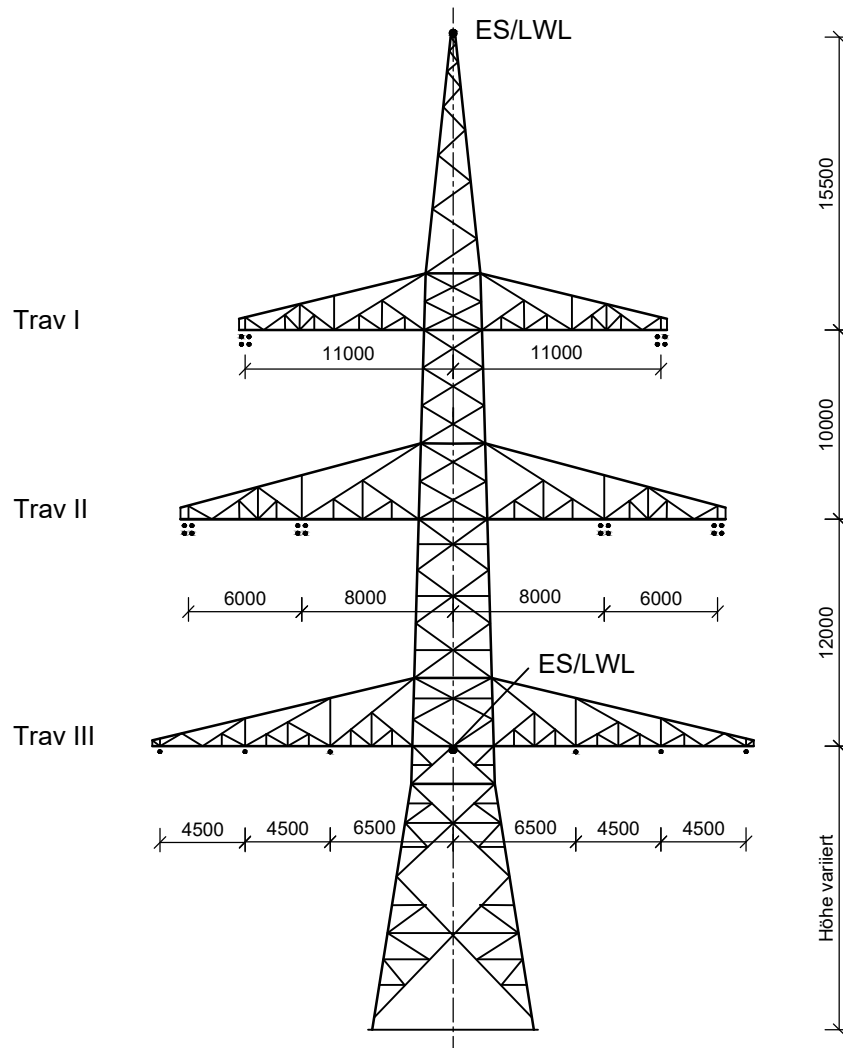
Winkelabspannmast WA160 ; DA-4-DE Ltg. Nr. B159: Mast-Nr. 10, 74, 75, 90
