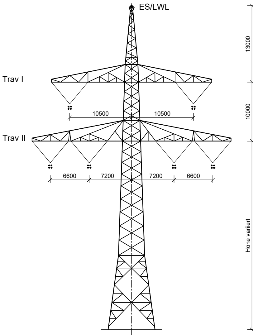
Tragmast T2; D-2-D
