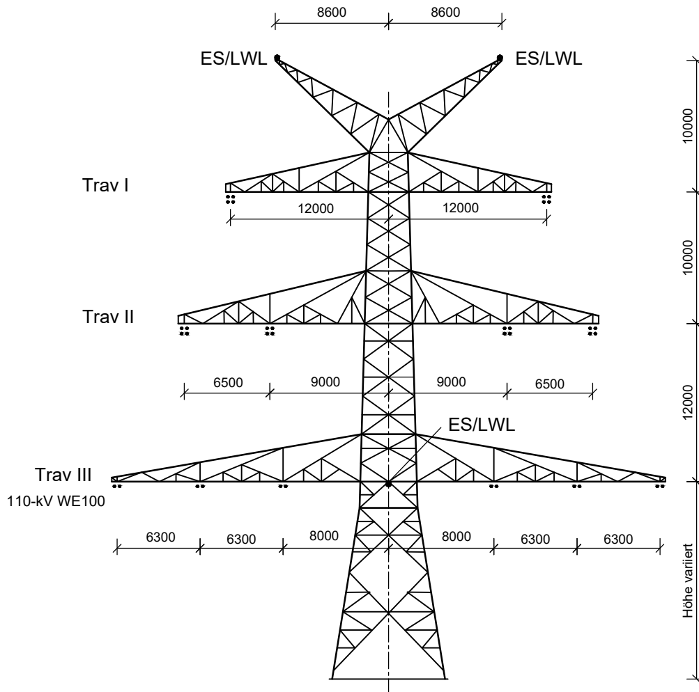
Winkelabspannmast WA140WAZ ; DA-4-DE Ltg. Nr. B159: Mast-Nr. 110
