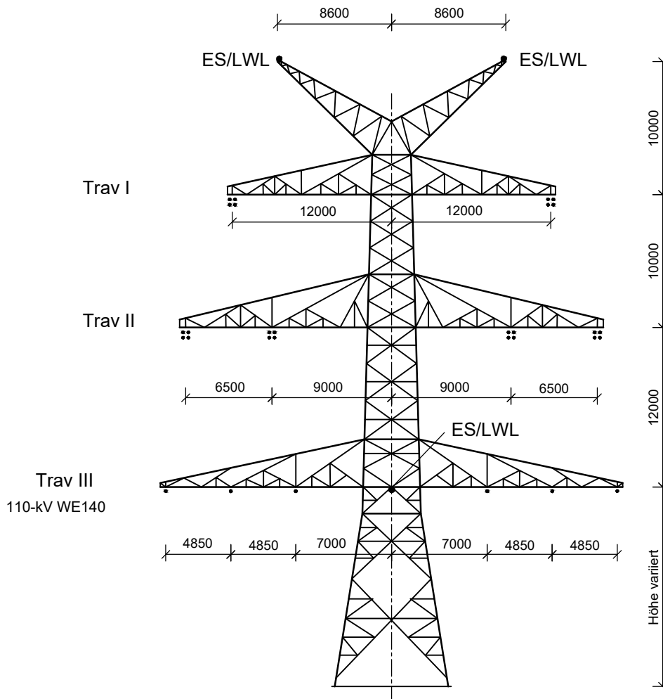
Winkelabspannmast WA140WAZ ; DA-4-DE Ltg. Nr. B159: Mast-Nr. xxx
