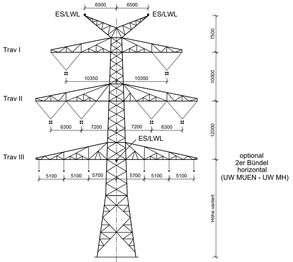
Tragmast T2; DA-4-DE
