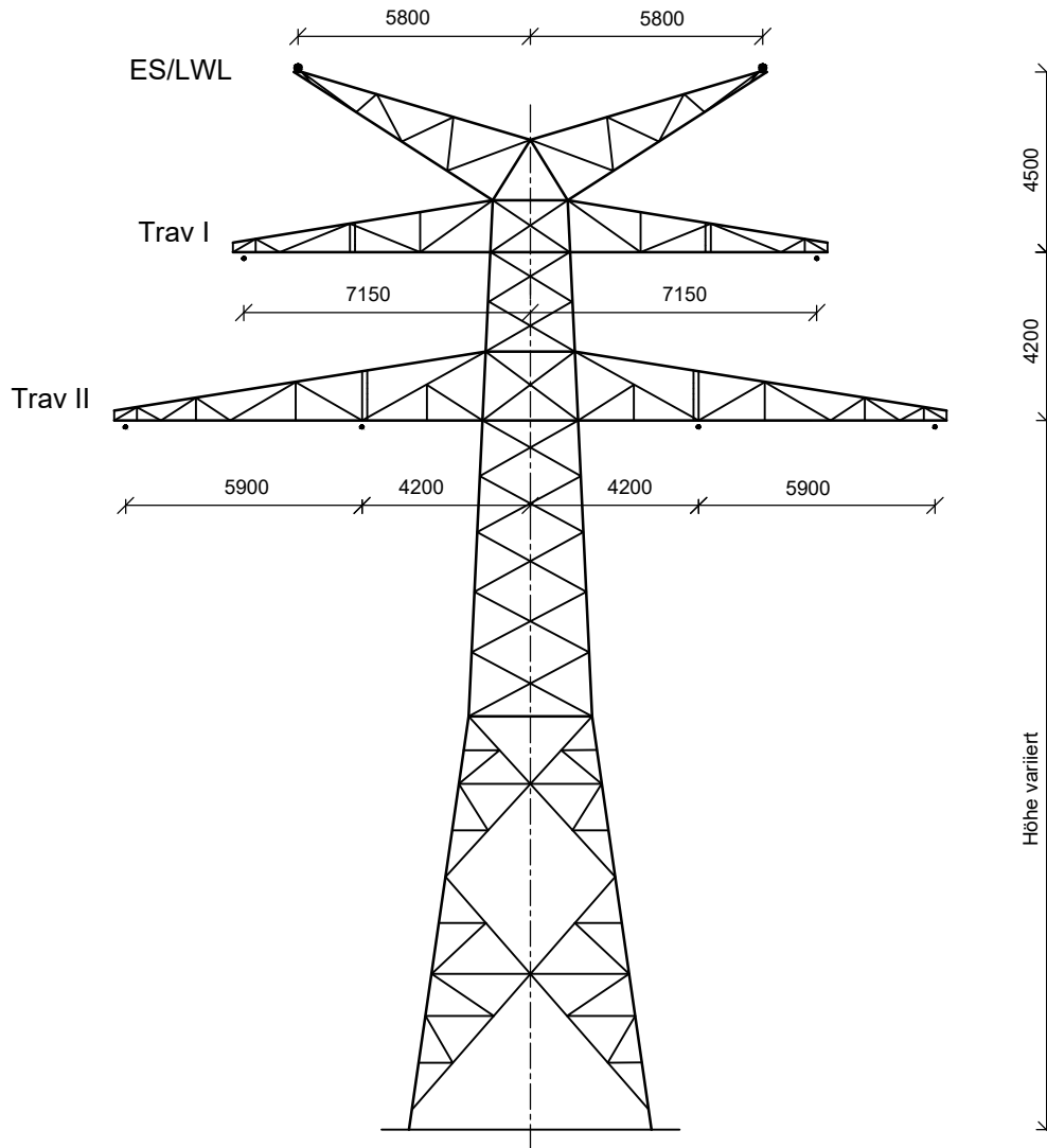
Winkelabspannmast WE/WAdiff/WA100 ; A-2-D Ltg. Nr. B159: Mast-Nr. 110A, 111A
