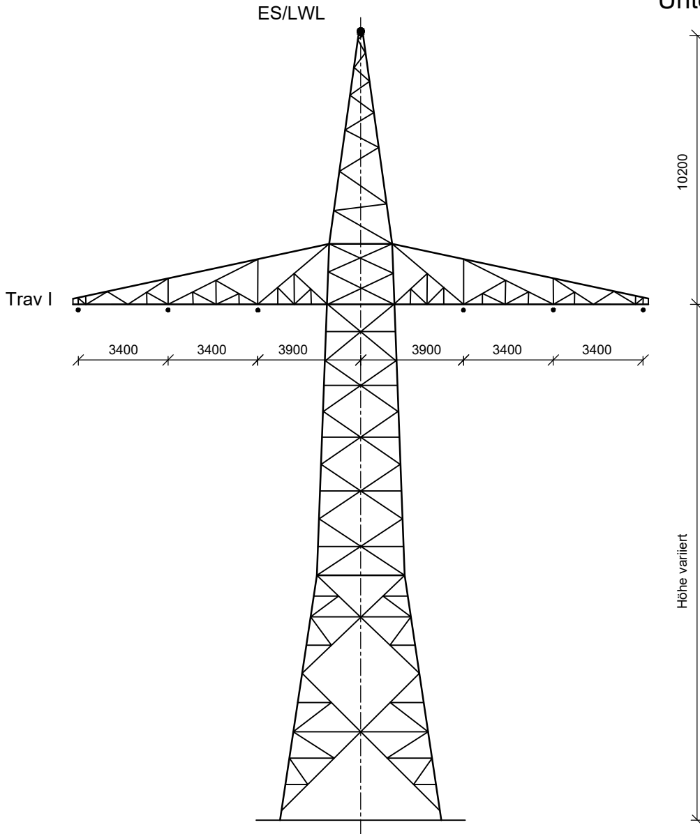
Winkelabspannmast WE/WAdiff/WA140 ; A-2-E Ltg. Nr. B159A: Mast-Nr. 1
