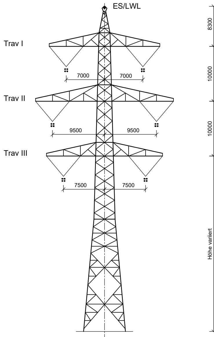
Tragmast T2; D-2-T Ltg. Nr. B159: Mast-Nr. 21
